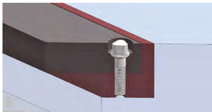
Bezpečnostní šroub
