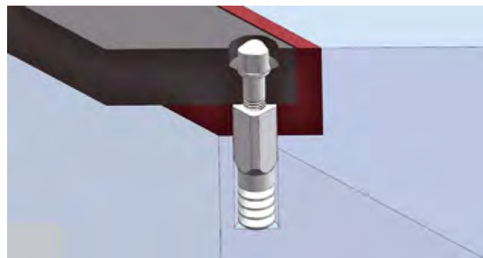
Bezpečnostní šroub + pouzdro s chemickou kotvou
