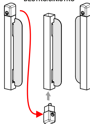
MONTAGGIO DESTRO/SINISTRO
